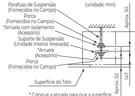
Fig. 3.7. Montagem Porcas e Arruela
