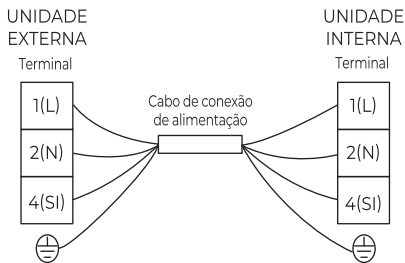
Diagrama da Fiação Elétrica
