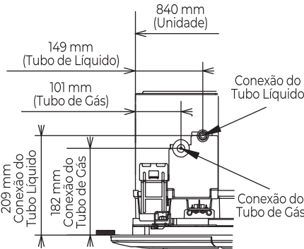
Fig. 4.1. Posição da Conexão da Tubulação
